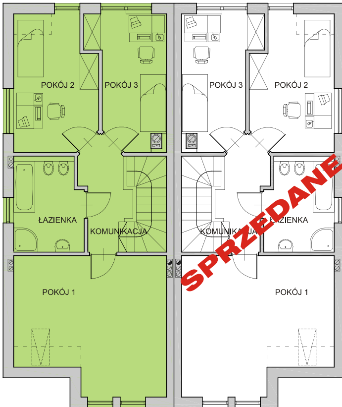
RZUT PIĘTRA
